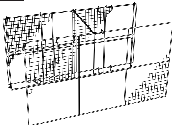
梱包時
